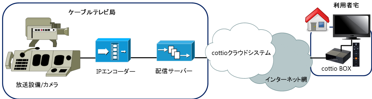
(図2) コミチャンライブ配信システム構成
